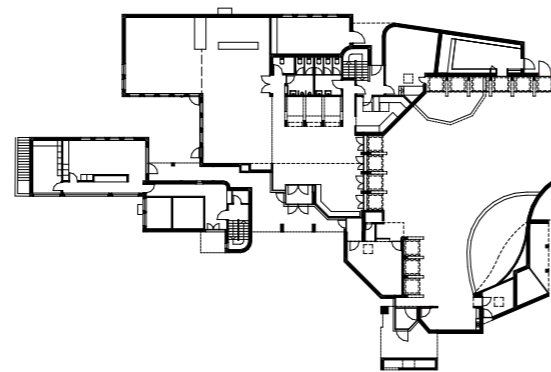
Grundriss Erdgeschoss
